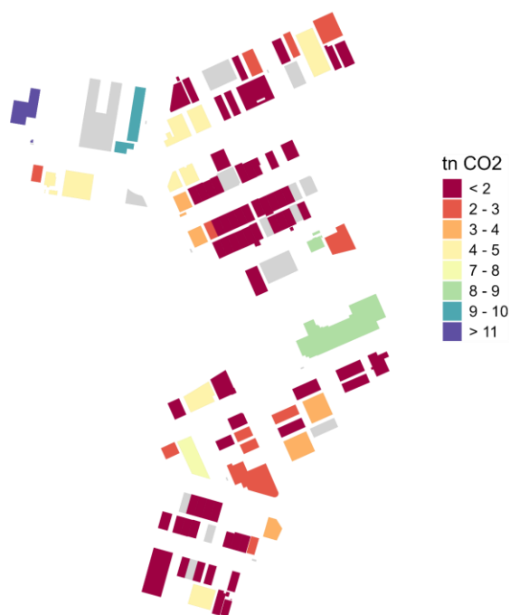
Figura 14. Emisiones anuales evitadas en los edificios con usos de tipo terciario, para el escenario con potencias instalables óptimas.
