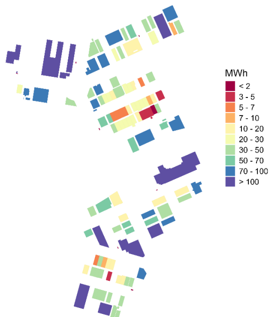
Figura 5. Producción fotovoltaica anual en todos los edificios del polígono, para el escenario con potencias instalables óptimas.
