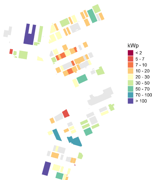
Figura 8. Potencia instalable óptima asignada a los edificios con usos de tipo industrial.
