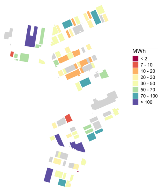
Figura 9. Producción fotovoltaica anual en los edificios con usos de tipo industrial.
