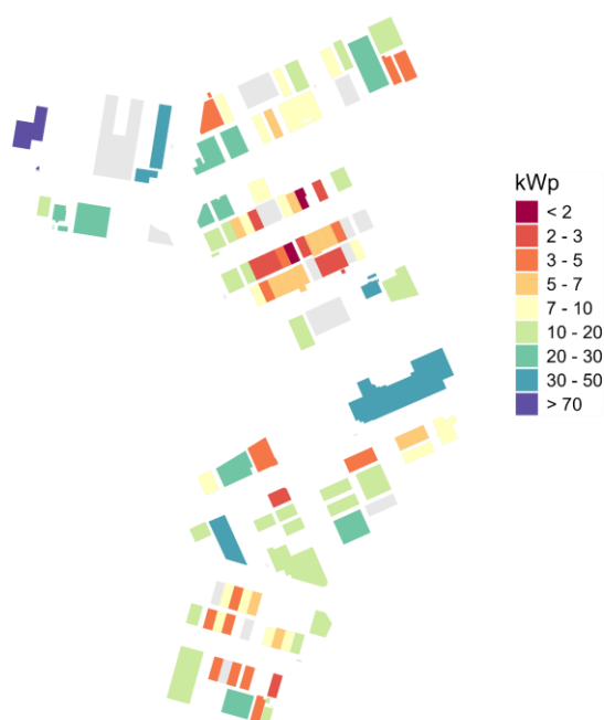
Figura 12. Potencia instalable óptima asignada a los edificios con usos de tipo terciario.
