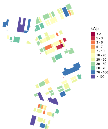
Figura 4. Potencia instalable óptima para todos los edificios del polígono.
