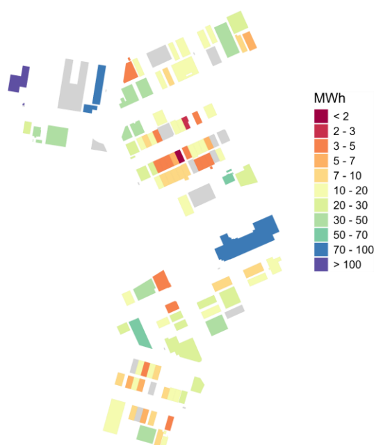
Figura 13. Producción fotovoltaica anual en los edificios con usos de tipo terciario, para el escenario con potencias instalables óptimas.
